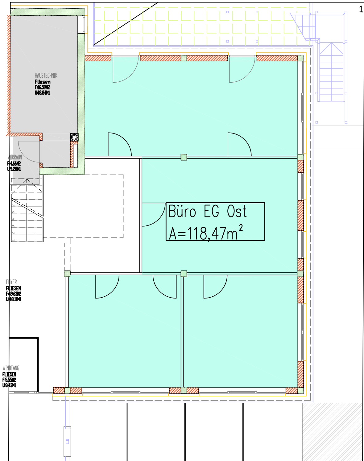
Büro EG OST A=118,47m 2
